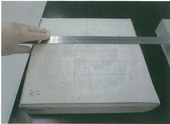
写真-1 試験体(グラウト面)
