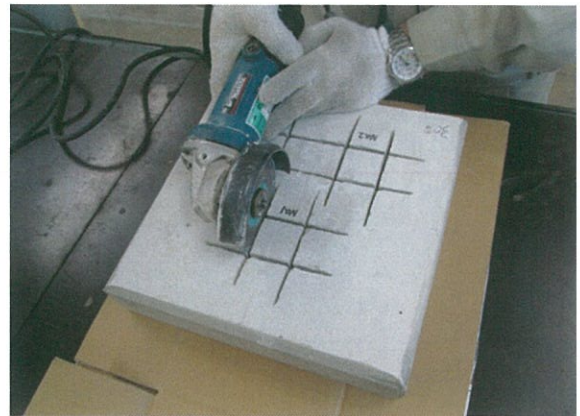
写真-2 40mm×40mm正方形の切り込み状況
